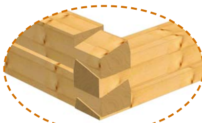
rybinový spoj s mezerou
